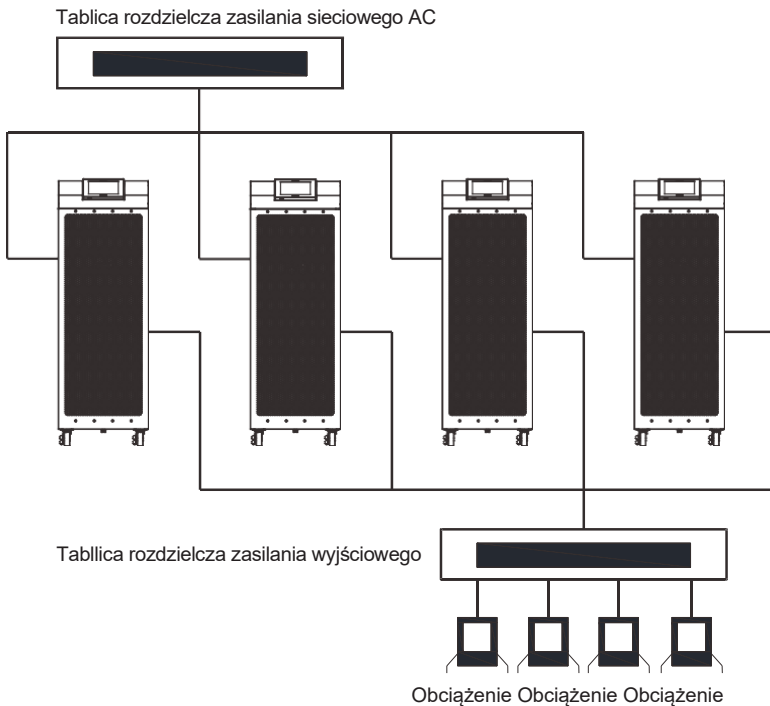
Rysunek 3-1: Konfiguracja równoległych UPS
