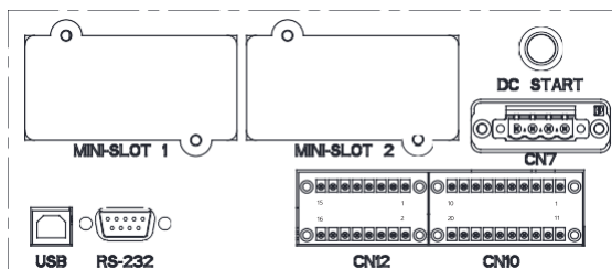
Rysunek 5-1: Interfejs komunikacyjny
