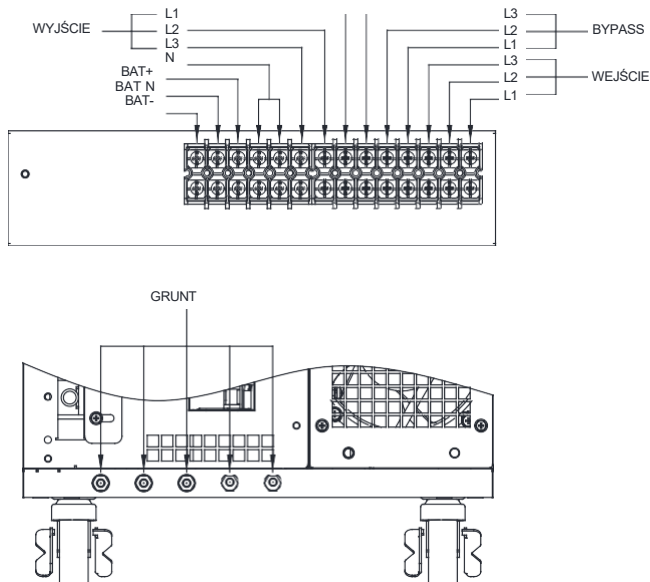
Rysunek 2-7: Schemat listwy zaciskowej modelu 20k BX
