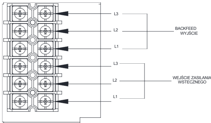
Rysunek 2-8: Listwa zaciskowa zasilania zwrotnego modelu VFI 20k TAP PF1 3/3 BX
