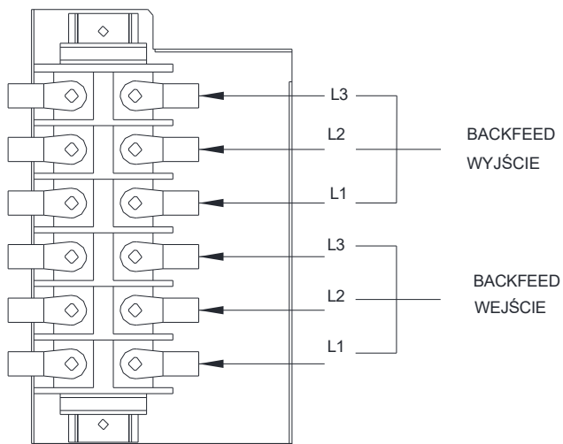
Rysunek 2-12: Listwa zaciskowa zasilania zwrotnego modeli VFI 60-80k TAP PF1 3/3 BX
