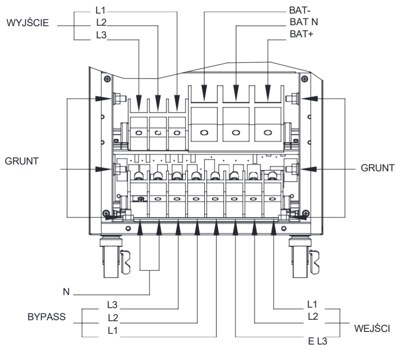
Rysunek 2-11: Schemat listwy zaciskowej modeli 60-80k BX
