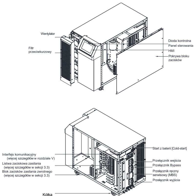
Rysunek 2-3: Schemat obudowy UPS VFI 20-40k TAP PF1 3/3 BX
