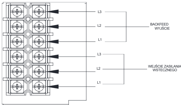
Rysunek 2-10: Listwa zaciskowa zasilania zwrotnego modelu VFI 30-40k TAP PF1 3/3 BX
