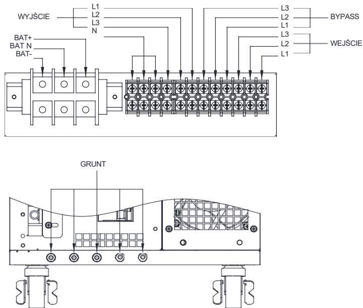
Rysunek 2-9: Schemat listwy zaciskowej modelu 30k/40k BX
