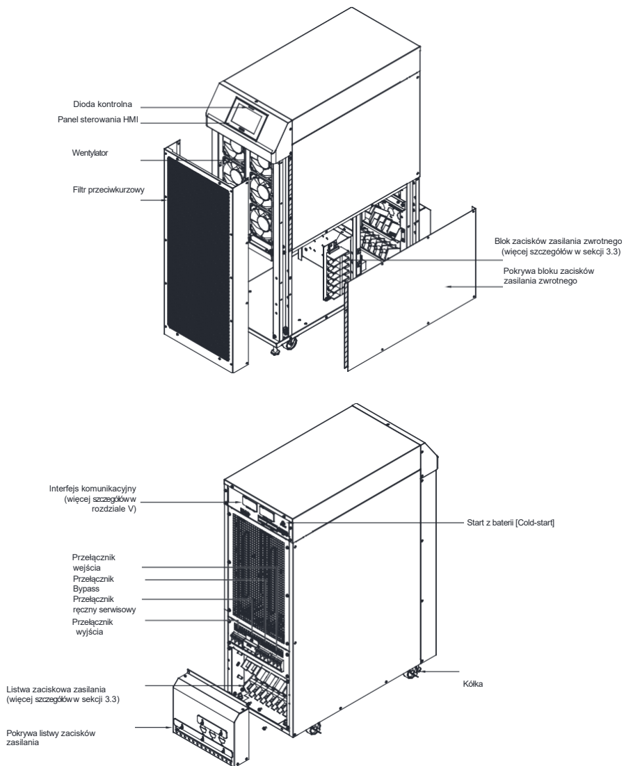
Rysunek 2-5: Schemat obudowy UPS VFI 60-80k TAP PF1 3/3 BX
