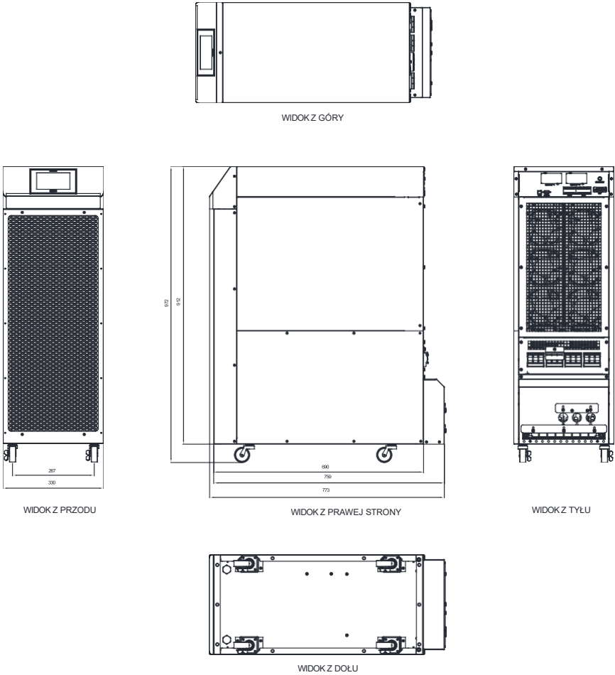
Rysunek 2-6: Schemat wymiarów obudowy UPS VFI 60-80k TAP PF1 3/3 BX
