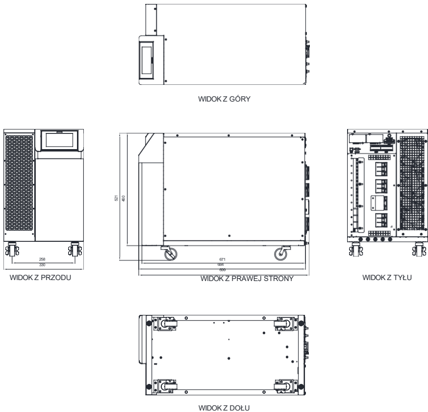
Rysunek 2-4: Schemat wymiarów obudowy UPS VFI 20-40k TAP PF1 3/3 BX
