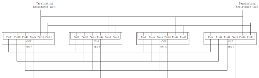
Rysunek 3-2: Schemat połączeń sekwencji równoległych UPS:
