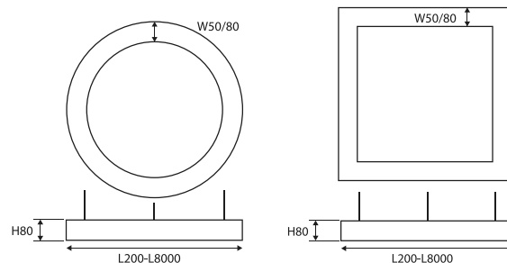
► Dostępne na zamówienie wymiary oprawy
