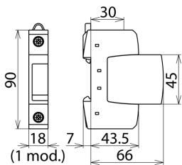
Rysunek wymiarowy DG S 275 VA
