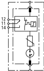
Schemat połączeń DG S 75 VA FM
