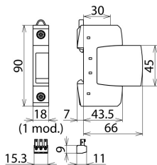
Rysunek wymiarowy DG S 275 VA FM
