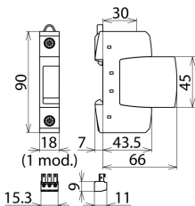
Rysunek wymiarowy DG S 385 VA FM
