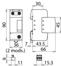
Rysunek wymiarowy DGP M 255 FM
