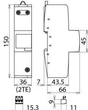
Rysunek wymiarowy DGPM 1 255 FM
