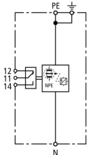
Schemat połączeń DGPM 1 255 FM
