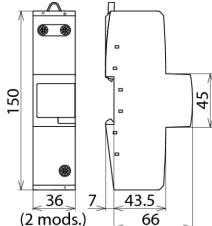
Rysunek wymiarowy DGPM 440
