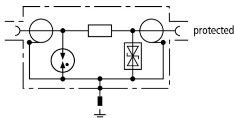
Schemat połączeń DGA BNC VCD
