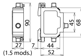
Rysunek wymiarowy DGA FF TV
