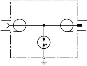
Schemat połączeń DGA G SMA
