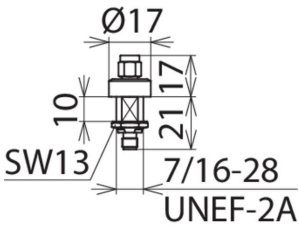
Rysunki wymiarowe DGA G SMA
