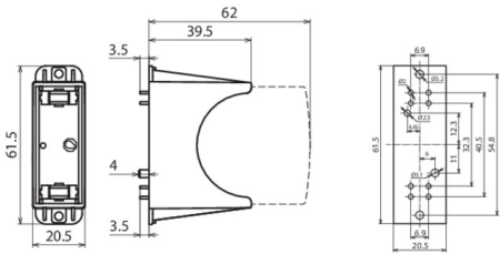
Rysunek wymiarowy DG PCB PV SCI 500
