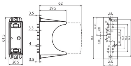
Rysunek wymiarowy DG PCB PV SCI 600 FM
