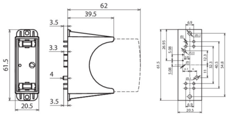
Rysunek wymiarowy DG PCB PV 300 FM
