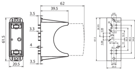
Rysunek wymiarowy DG PCB PV 500 FM
