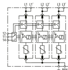
Schemat połączeń DG MP TNC ACI 275 FM
