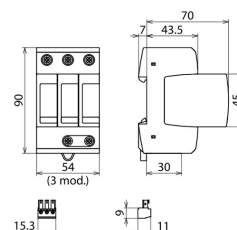
Rysunek wymiarowy DG MP TNC ACI 275 FM
