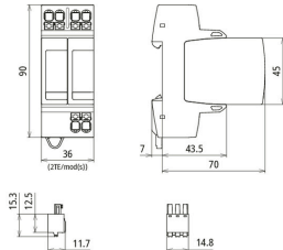
Rysunek wymiarowy DG MP TT 2P ACI 275 FM
