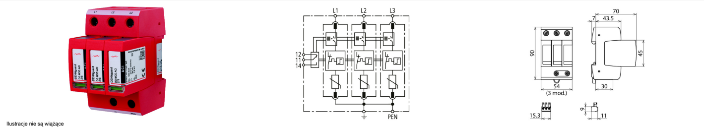
Ilustracje nie są wiążące Schemat połączeń DG M TNC ACI 275 FM Rysunek wymiarowy DG M TNC ACI 275 FM
