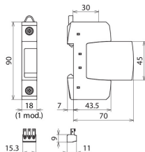
Rysunek wymiarowy DG S ACI 275 FM
