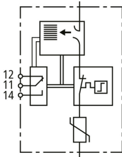
Schemat połączeń DG S ACI 275 FM
