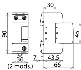
Rysunek wymiarowy DB M 1 150
