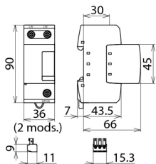
Rysunek wymiarowy DB M 1 150 FM
