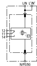
Schemat połączeń DB M 1 150 FM
