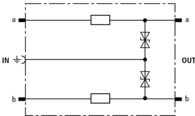
Schemat połączeń DRL RE 12
