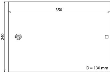
Rysunek wymiarowy DPG LSA 60 P
