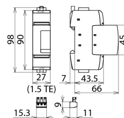
Rysunek wymiarowy DG SE DC 550 FM
