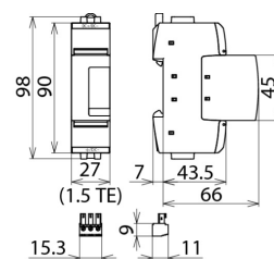
Rysunek wymiarowy DG SE DC 900 FM
