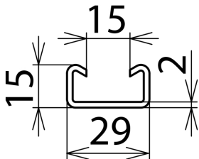
Rysunek wymiarowy AS SAK 1000 V2A
