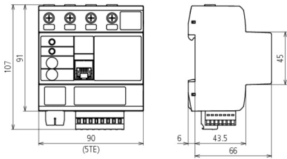
Rysunek wymiarowy DRC SD 1 1
