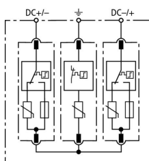
Schemat połączeń DG M YPV SCI 150
