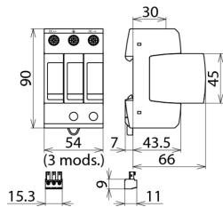
Rysunek wymiarowy DG M YPV SCI 1000 FM
