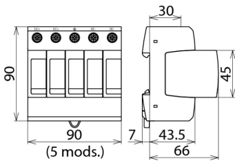
Rysunek wymiarowy DG M PV2 SCI 1000
