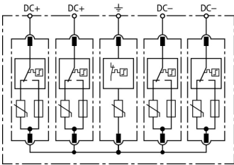
Schemat połączeń DG M PV2 SCI 1000
