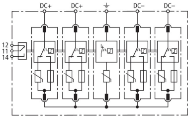
Schemat połączeń DG M PV2 SCI 1000 FM
