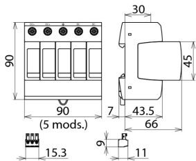
Rysunek wymiarowy DG M PV2 SCI 1000 FM
