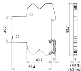
Rysunek wymiarowy BCO CL2 B 180
