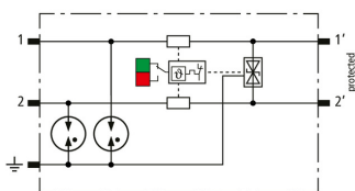
Schemat połączeń BCO CL2 BE HF 5
