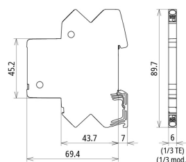
Rysunek wymiarowy BCO CL2 BE HF 5
