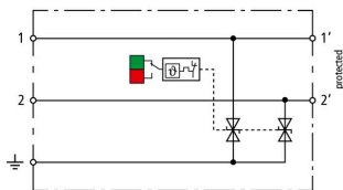
Schemat połączeń BCO CL2 BE 48
