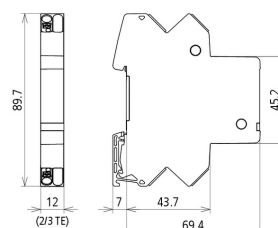
Rysunek wymiarowy BCO CL2 BD HC10A 24
