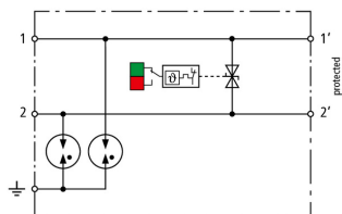
Schemat połączeń BCO CL2 BD HC10A 24
