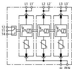
Schemat połączeń DG MP TNC 275 FM
