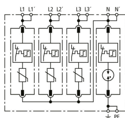
Schemat połączeń DG MP TT 275
