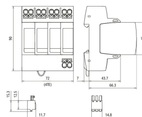
Rysunek wymiarowy DG MP TT 275 FM
