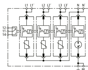
Schemat połączeń DG MP TT 275 FM
