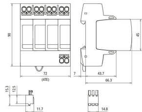
Rysunek wymiarowy DG MP TT 320 FM
