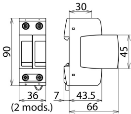
Rysunek wymiarowy DG MP TN 275 FM
