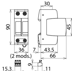
Rysunek wymiarowy DG MP TT 2P 275
