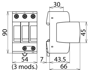
Rysunek wymiarowy DG M TNC 385
