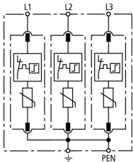
Schemat połączeń DG M TNC 385
