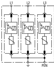
Schemat połączeń DG M TNC 440
