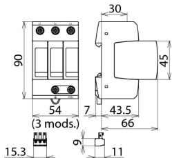
Rysunek wymiarowy DG M TNC 275 FM
