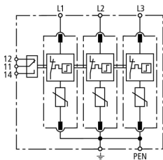
Schemat połączeń DG M TNC 275 FM
