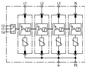
Schemat połączeń DG M TNS 150 FM
