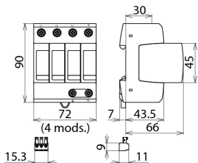
Rysunek wymiarowy DG M TNS 385 FM
