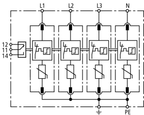
Schemat połączeń DG M TNS 385 FM
