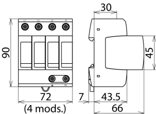
Rysunek wymiarowy DG M TT 150
