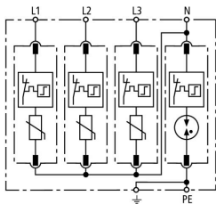
Schemat połączeń DG M TT 150
