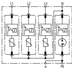
Schemat połączeń DG M TT 275
